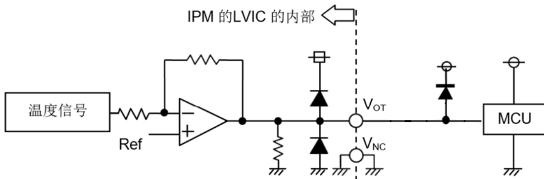
图 6.2: VOT 输出电路
