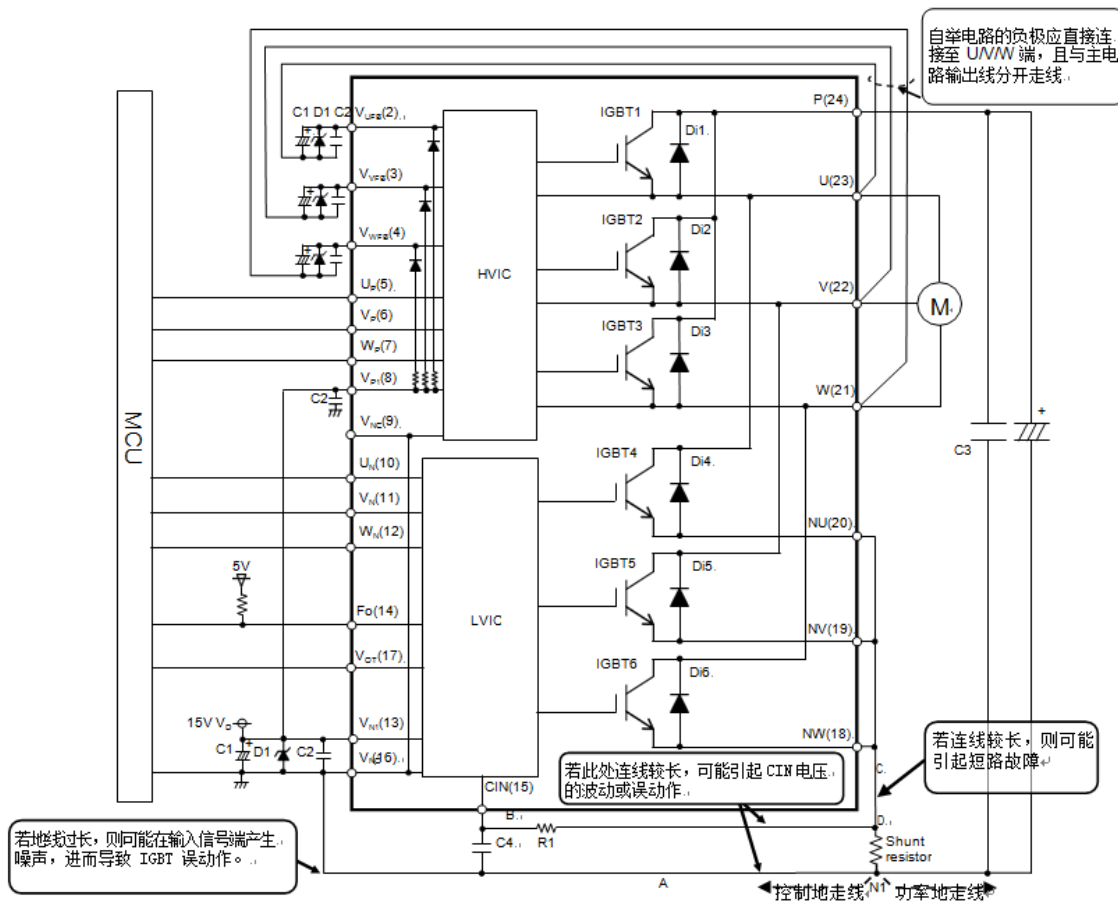
图 13: 典型应用电路
