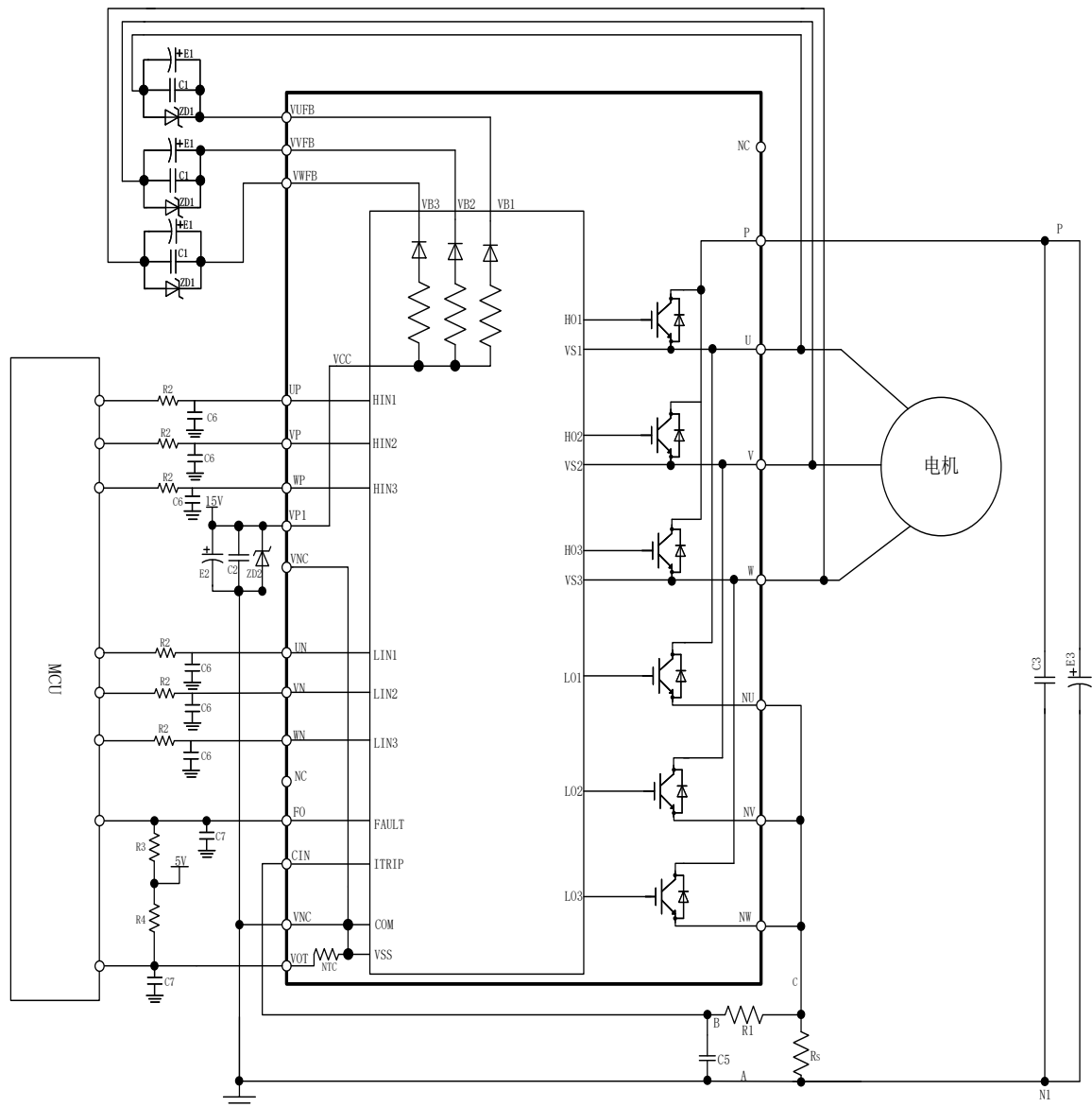
图 16: 典型应用电路
