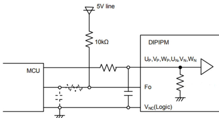
图 14: 推荐的 MCU 输入输出接口电路
