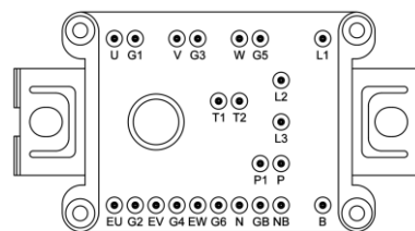
引脚示意图
